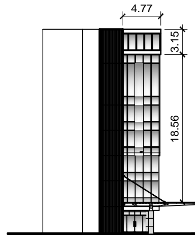
② ELEVACION LATERAL DERECHA MURO CORTINA
