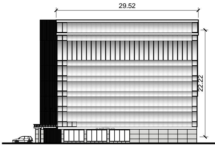
① ELEVACION FRONTAL MURO CORTINA
