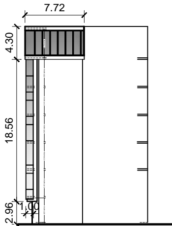
③ ELEVACION LATERAL IZQUIERDA MURO CORTINA
