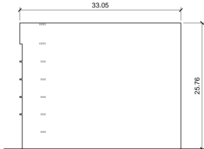
② ELEVACION LATERAL DERECHA MURO CORTINA
